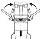
Abb. 12: Verschlusshebel öffnen
