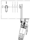
Abb. 4: Lasttrennschalter in I-Stellung, Ausziehen nicht möglich
