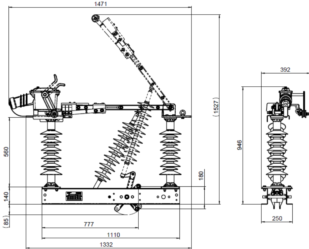
Fig. 3: Dimensions FHV-B3-25/S
