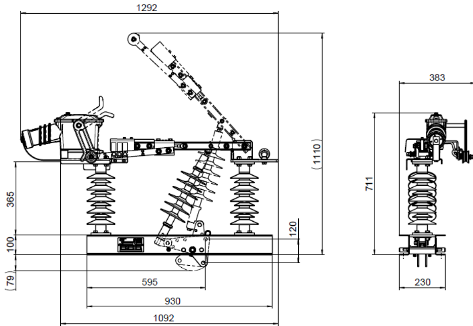
Fig. 2: Dimensions FHV-B3-15/S
